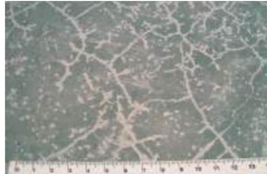
Kuruma rötresi sonucu erken yaş çatlakları
